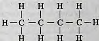
n -Butane
