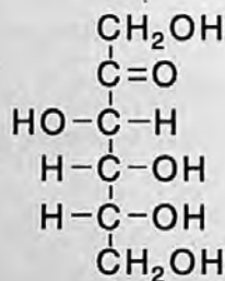
Fructose
